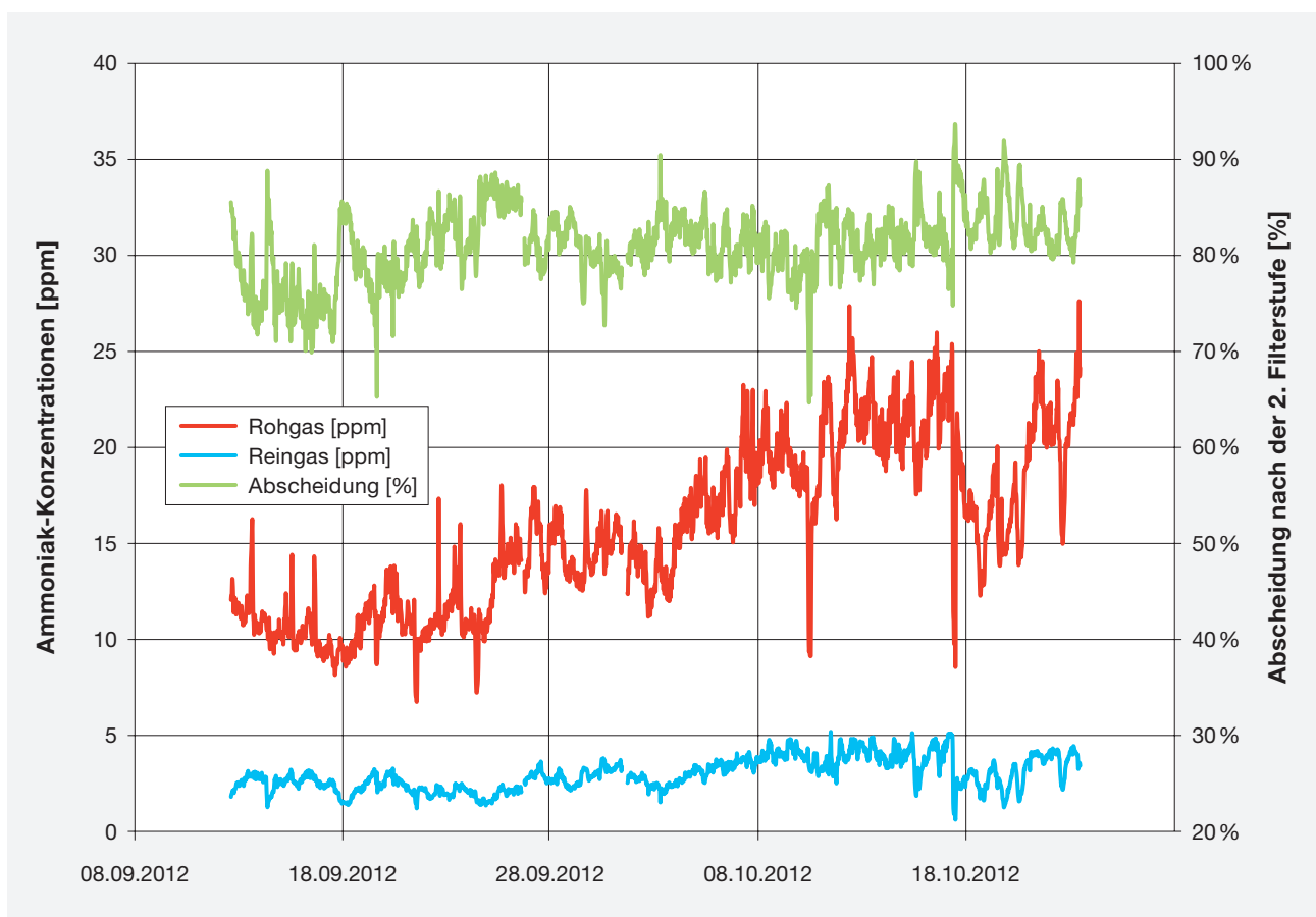
Bild 4: Abscheidegrad und Verlauf der Ammoniak-Konzentrationen im Roh- und Reingas während der Sommermessung
