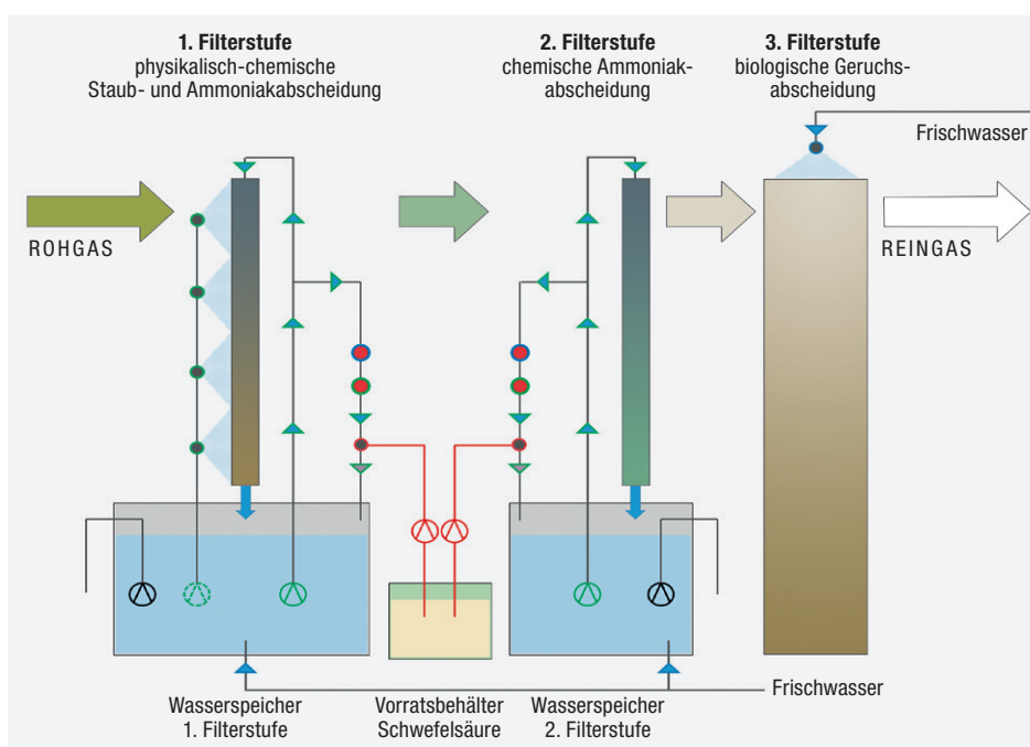
Bild 2: Schematische Darstellung des Funktionsprinzips
