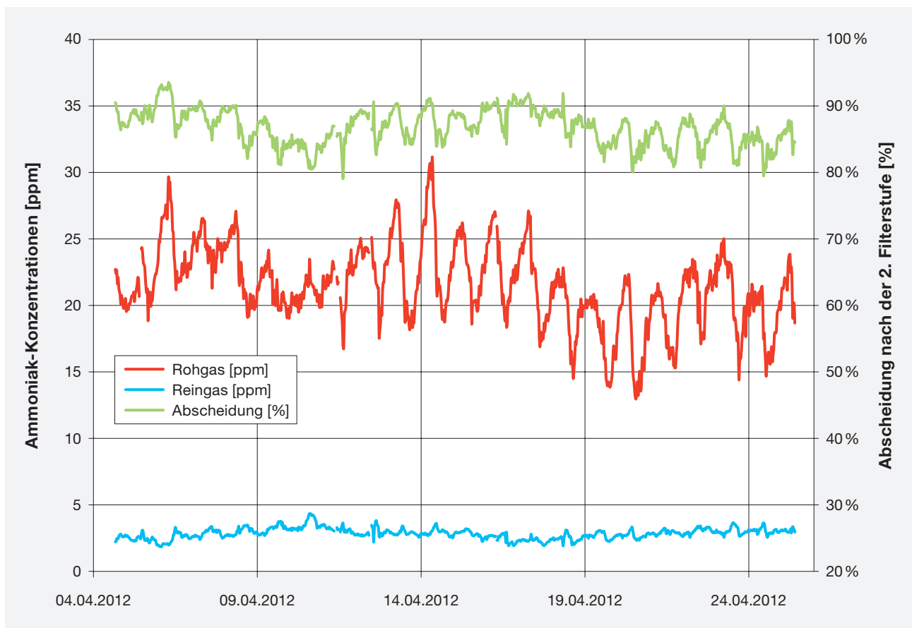
Bild 3: Abscheidegrad und Verlauf der Ammoniak-Konzentrationen im Roh- und Reingas während der Wintermessung
