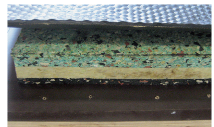
Bild 3: Aufbau der Gel-Matratze
