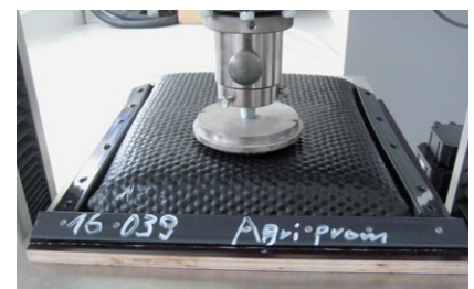
Bild 4: Messung der Verformbarkeit
