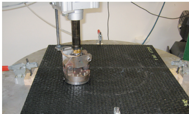
Bild 3: Dauertrittbelastung
