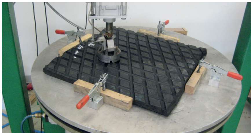
Bild 5: Dauertrittbelastung
