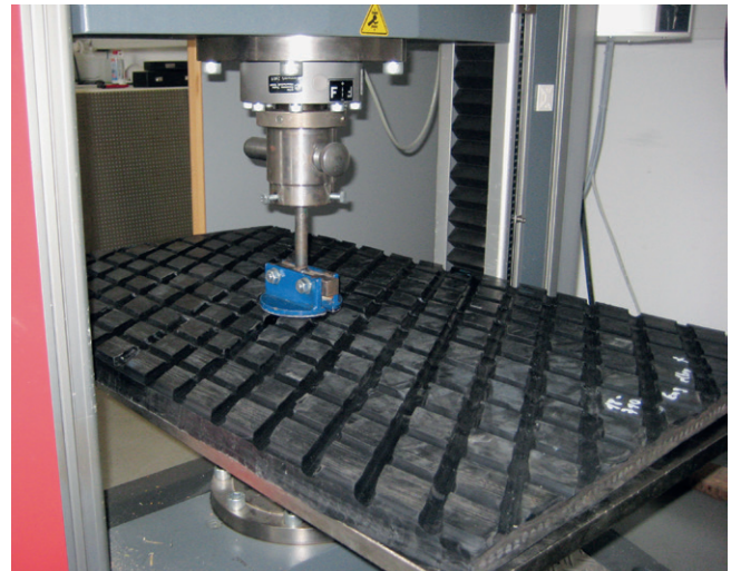
Bild 3: Messung der Verformbarkeit mit „künstlichem Kuhfuß“
