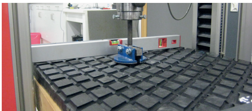
Bild 6: Messung Biegefestigkeit
