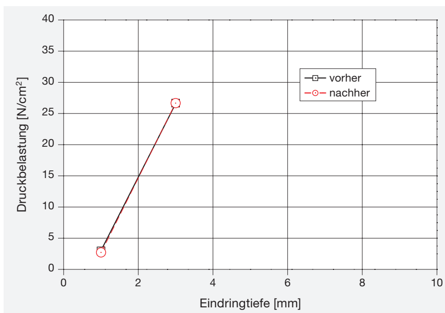
Bild 4: Verformbarkeit in Abhängigkeit vom Auflagedruck vor und nach der Dauertrittbelastung
