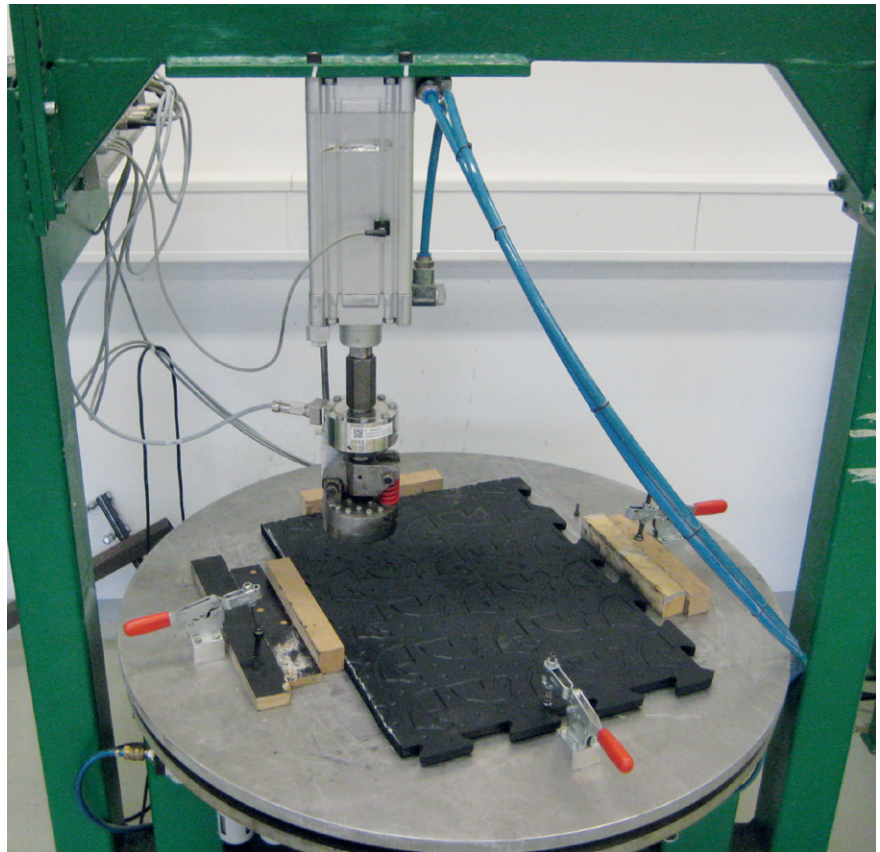
Bild 3: Dauertrittbelastung
