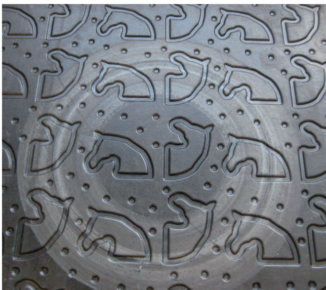
Bild 4: Oberseite Bodenbelag – nach der Dauertrittbelastung
