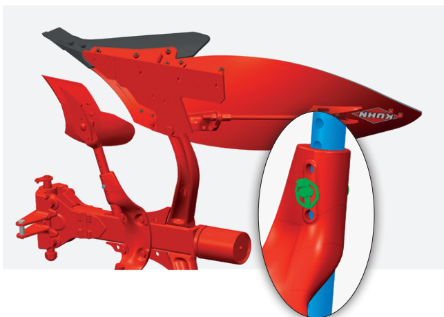
Bild 2: Vorschälereinstellung 3D-SKIM
