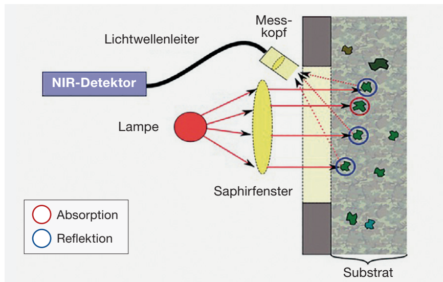
Bild 2: Funktionsprinzip und Systemaufbau „ZUNHAMMER VAN Control dual“
