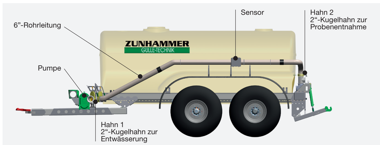
Bild 3: Schematischer Aufbau des DLG-Messsystems
