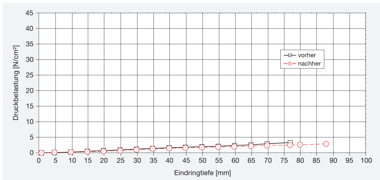
Bild 3: Verformbarkeit, Eindringtiefe der Kalotte ( r = 120 \text{ mm} ) in Abhängigkeit vom Auflagedruck
