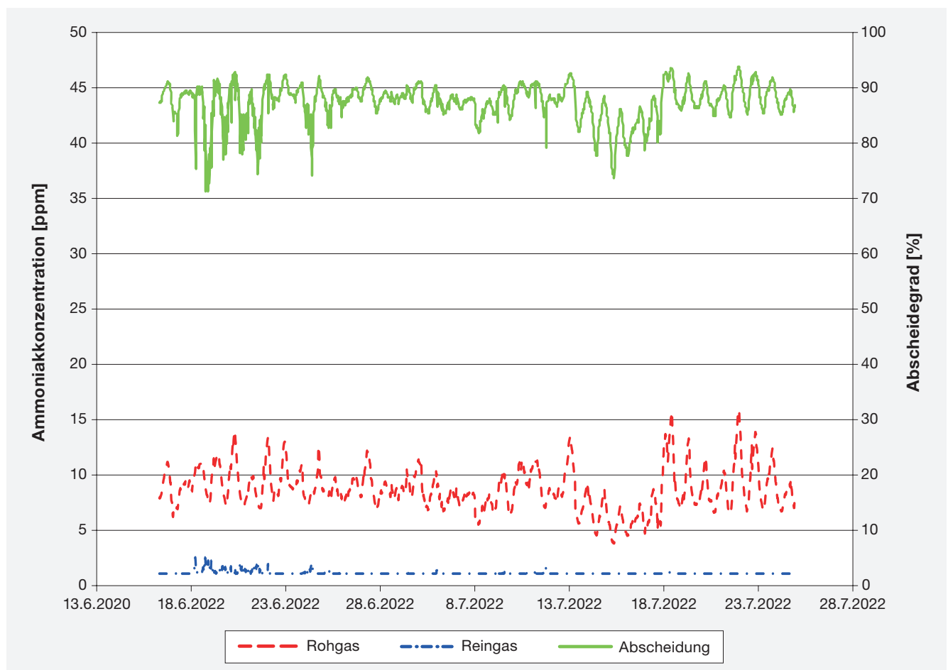
Bild 3: Abscheidegrad und Verlauf der Ammoniakkonzentrationen im Roh- und Reingas (Sommermessphase)
