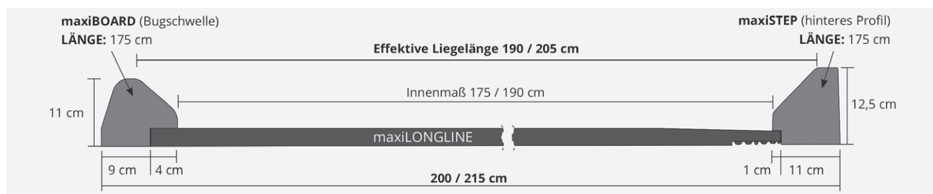
Bild 2: Systemskizze maxiBOX
