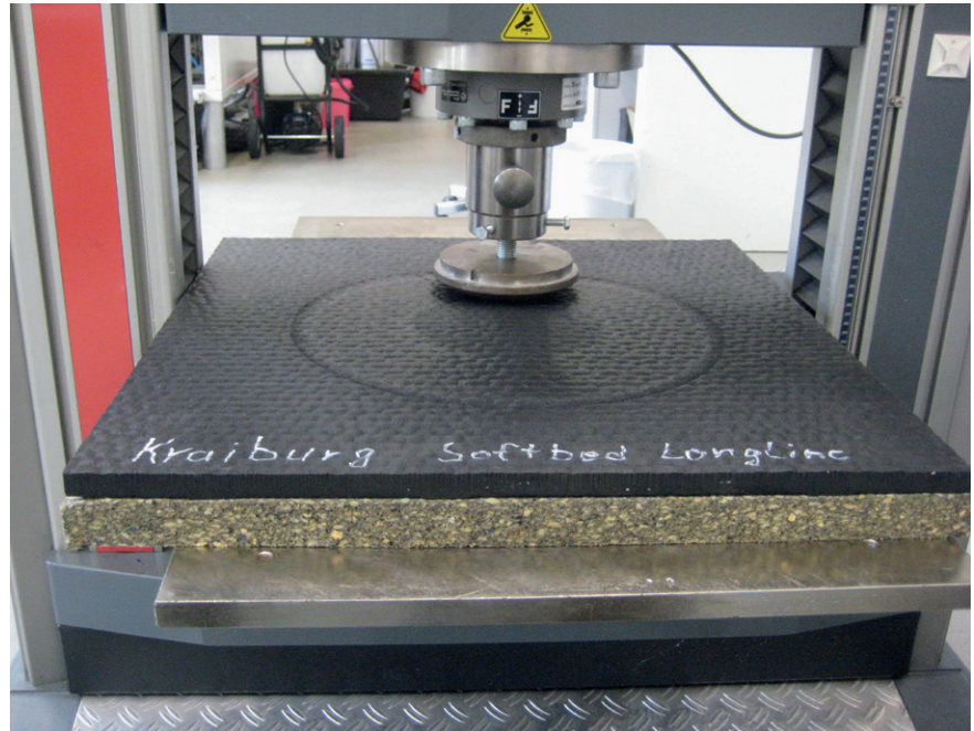
Bild 2: Messung Verformbarkeit
