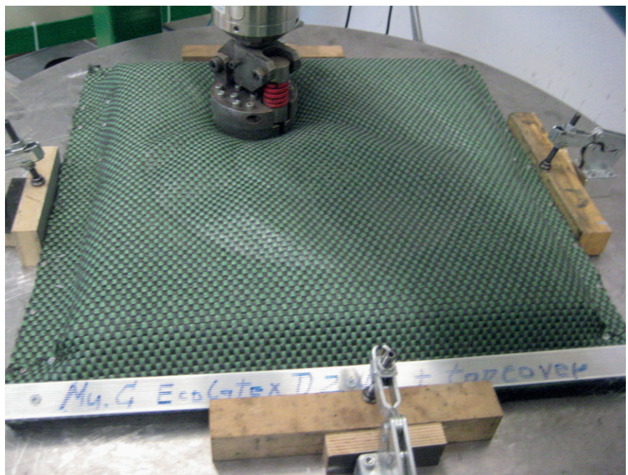
Bilder 2 und 3: Messung Verformbarkeit und Dauertrittbelastung
