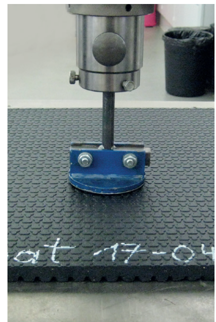
Bild 4: Messung der Verformbarkeit
