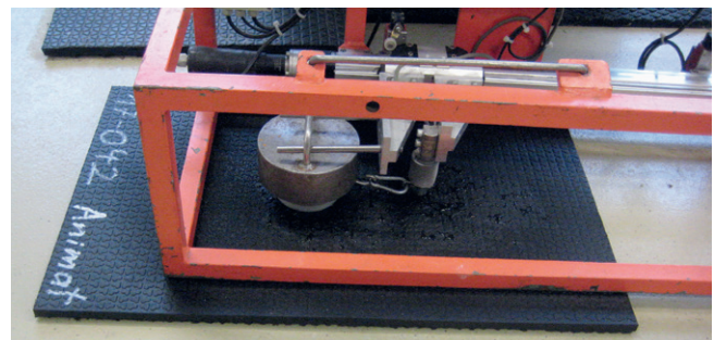
Bild 2: Messung der Rutschfestigkeit
