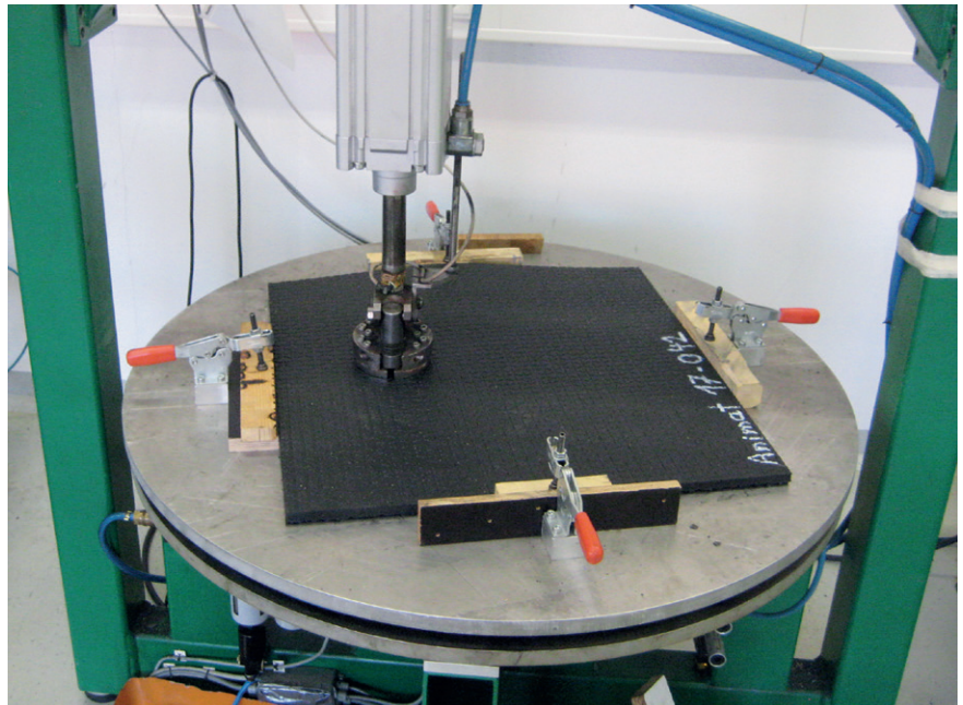
Bild 5: Dauertrittbelastung
