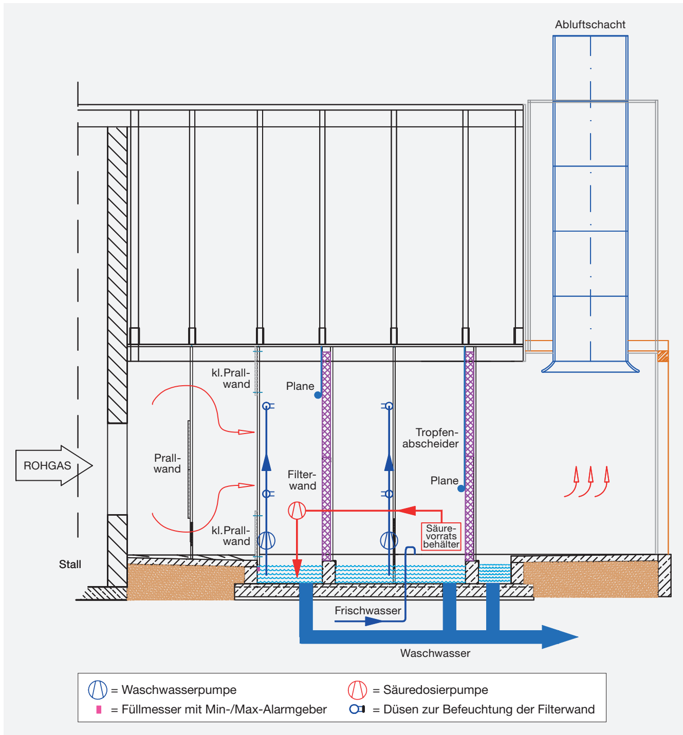
Bild 2: Schematische Darstellung des 1-stufigen Chemowäschers ASA-S1 im Saugprinzip
