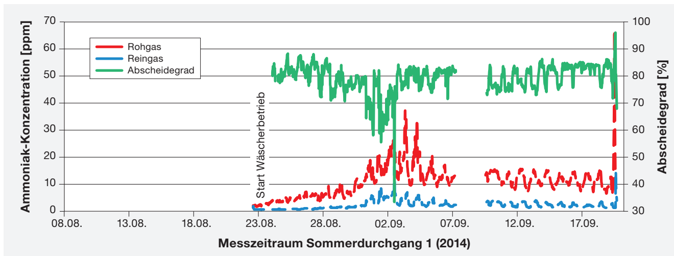
Bilder 3 und 4: Abscheidegrad und Verlauf der Ammoniak-Konzentration im Roh- und Reingas
