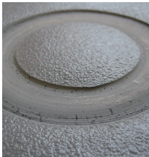
Bild 4: Testmuster nach dem Abriebtest
