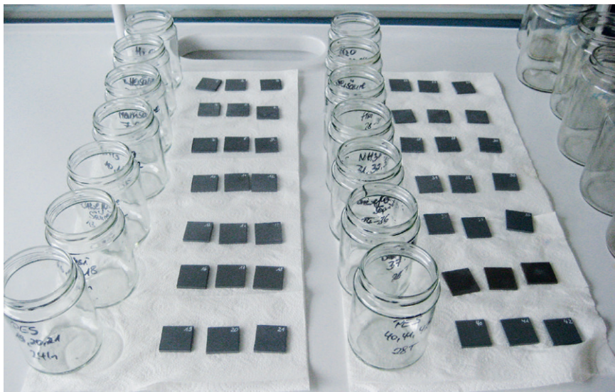
Bild 6: Prüfmuster nach Test Säurebeständigkeit
