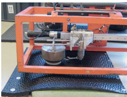
Bild 4: Messung der Rutschfestigkeit
