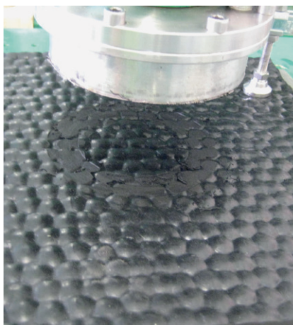
Bild 3: Testmuster nach Abriebtest
