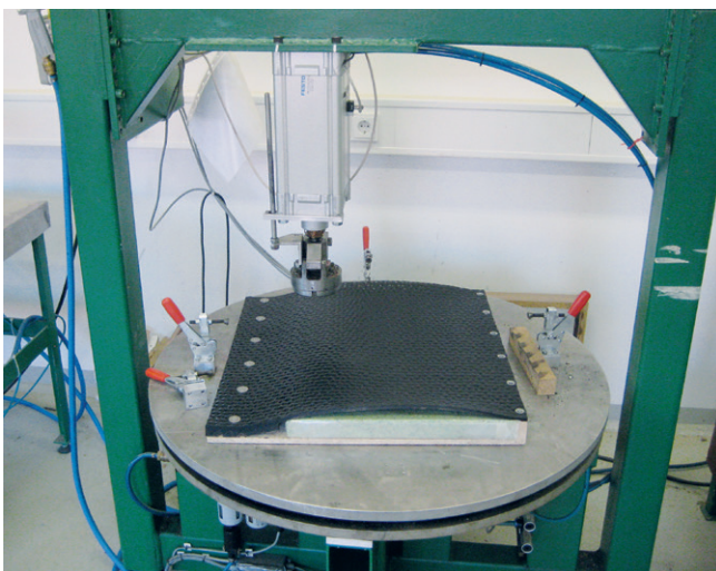
Bild 2: Dauertrittbelastung
