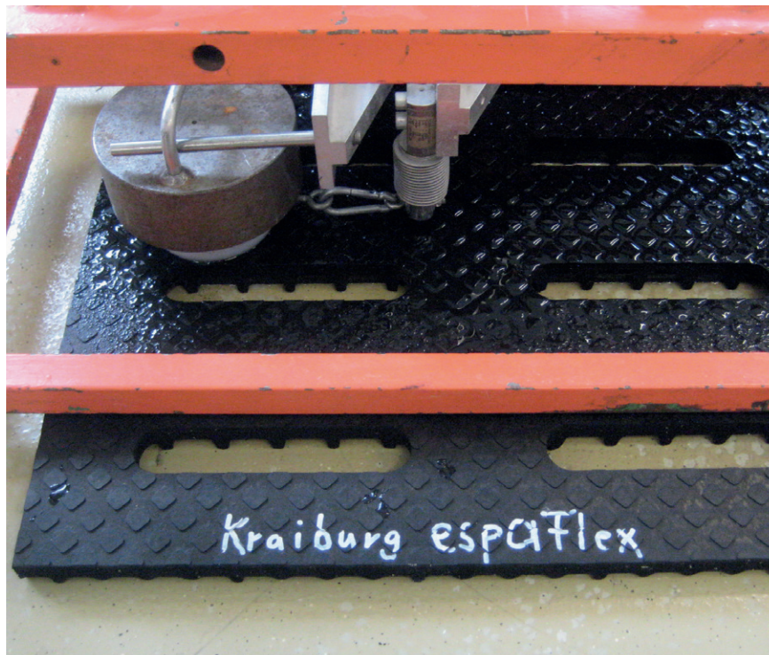
Bild 4: Messung der Rutschfestigkeit
