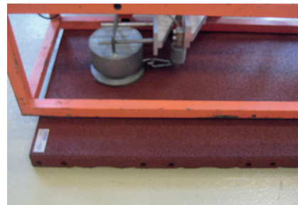
Bild 3: Messung der Rutschfestigkeit
