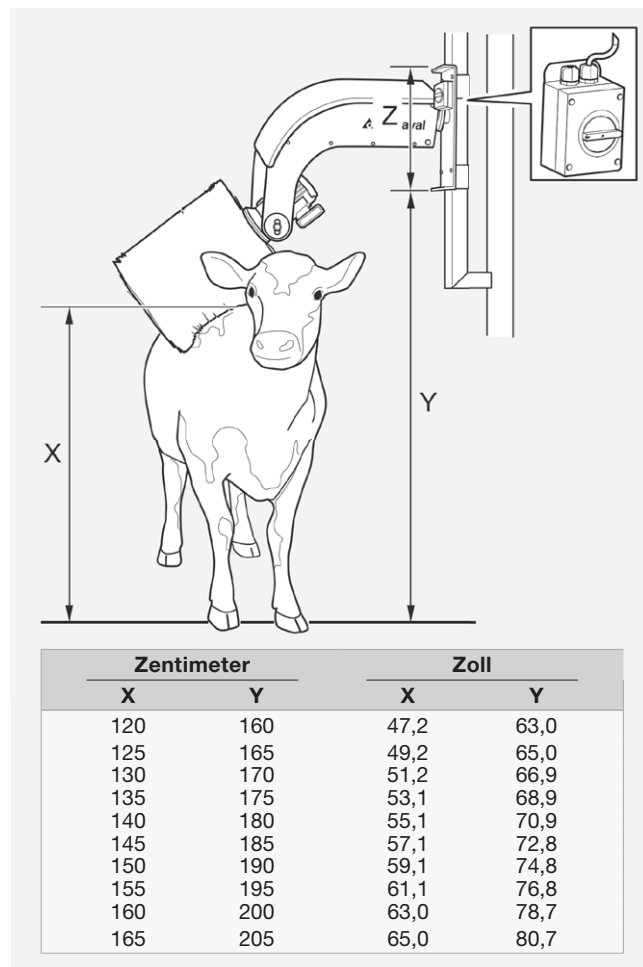
Bild 3: Ermittlung der Montagehöhe der Kuhputzmaschine
