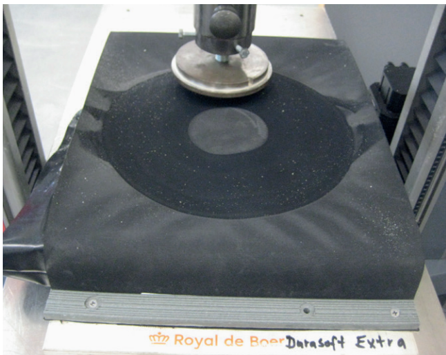
Bild 3: Messung der Verformbarkeit
