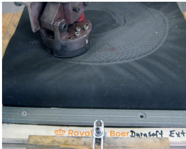
Bild 4: Dauertrittbelastung
