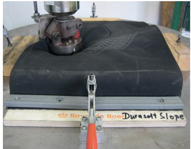
Bild 4: Dauertrittbelastung
