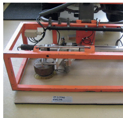
Bild 4: Messung der Rutschfestigkeit
