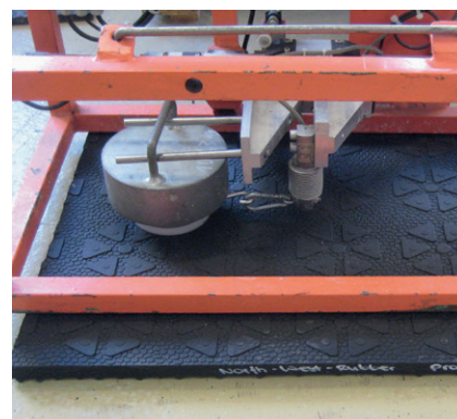
Bild 4: Messung der Rutschfestigkeit
