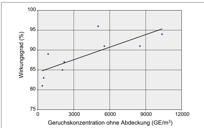
Bild 1: Wirkungsgrad des Abdecksystems Hexa-Cover auf Schweinegülle
