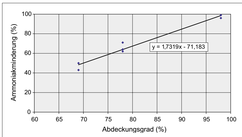
Bild 2: Minderung der Ammoniakemission
