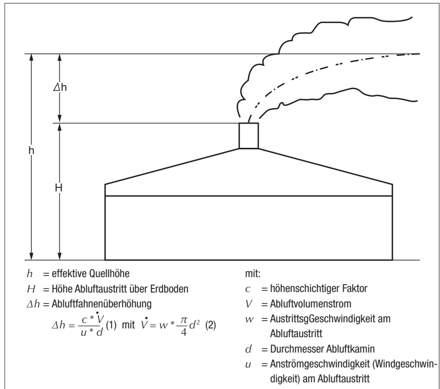
Bild 9: Schematische Darstellung und Berechnung der Abluftfahnenüberhöhung nach VDI 3471/3472 „Emissionsminderung; Tierhaltung – Schweine/Hühner“
