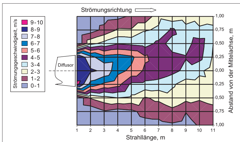
Bild 4: Profil der Abluftaustrittsströmung – Abluftkaminsystem mit Nachleitrad bei 230 V Betriebsspannung
