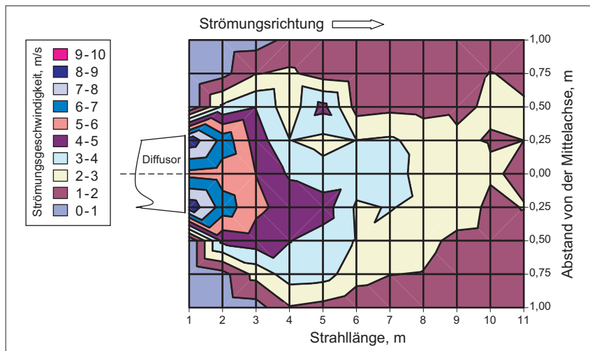
Bild 3: Profil der Abluftaustrittsströmung – Abluftkaminsystem ohne Nachleitrad bei 230 V Betriebsspannung
