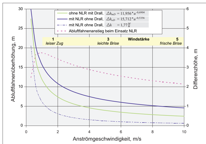
Bild 10: Abluftfahnenüberhöhung bis 10 m/s Anströmgeschwindigkeit – Abluftkaminsystem bei 230 V Betriebsspannung und 10 Pa Widerstand des angenommenen Lüftungssystems
