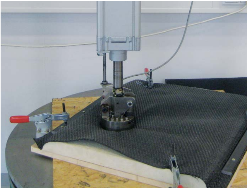
Bild 3: Dauertrittbelastung
